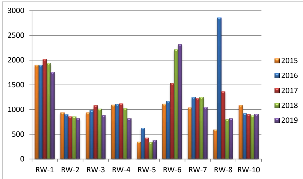
الشكل رقم (3-11): المعدلات السنوية لدرجة الملوحة (EC µS/cm) في مياه السدود خلال الأعوام (2019-2015)
