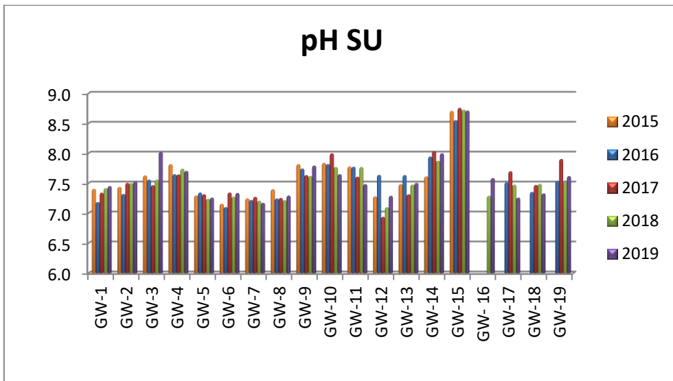
الشكل رقم (2-17): المعدلات السنوية لدرجة الحموضة (pH SU) في مواقع المياه الجوفية الخام خلال الأعوام (2015-2019)
