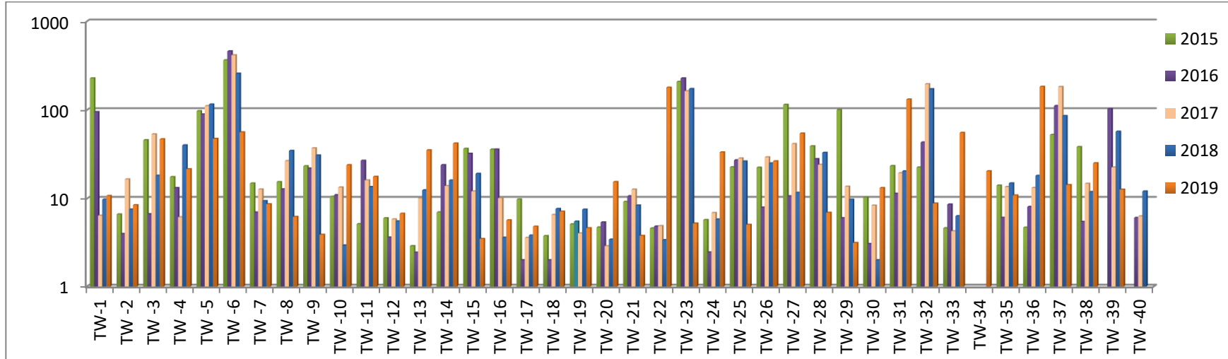
الشكل رقم (6-32): المعدلات السنوية لتركيز الأكسجين المستهلك حيويًا (BOD 5 mg/L) في محطات التنقية خلال الأعوام (2015-2019)
