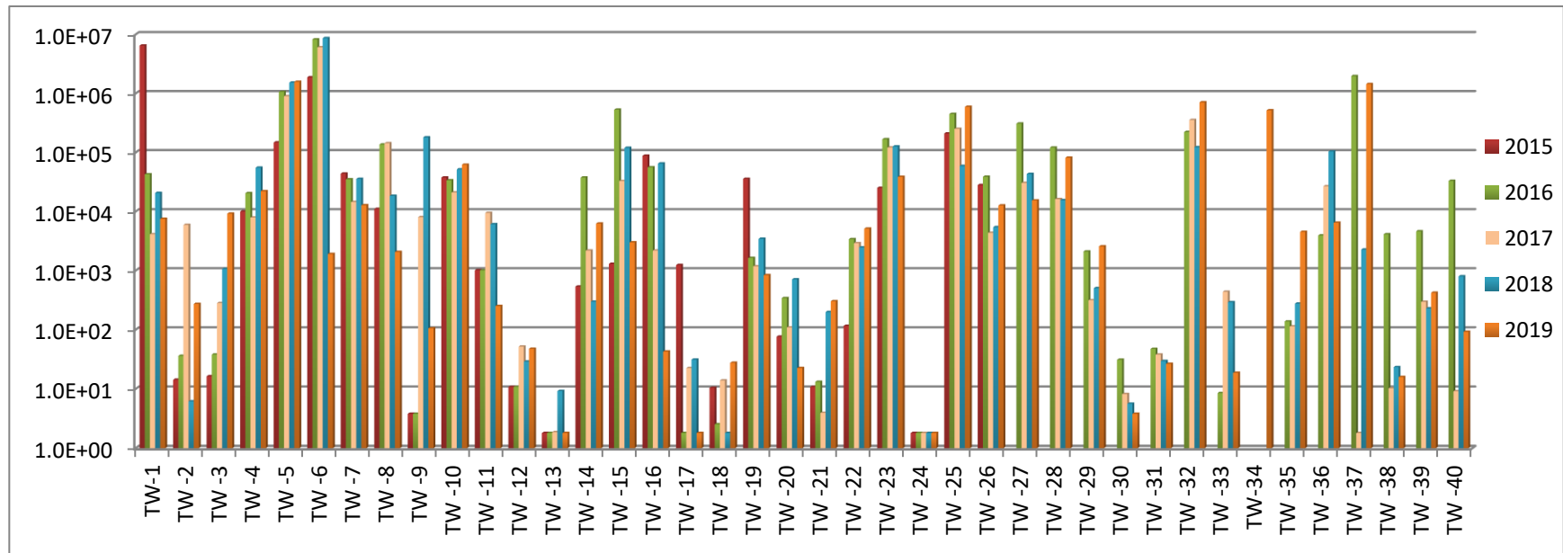
الشكل رقم (6-34): المعدلات الهندسية السنوية لأعداد الإشيرشيا القولونية ( E.coli MPN/100ml) في مواقع محطات التنقية خلال الأعوام (2019-2015)
