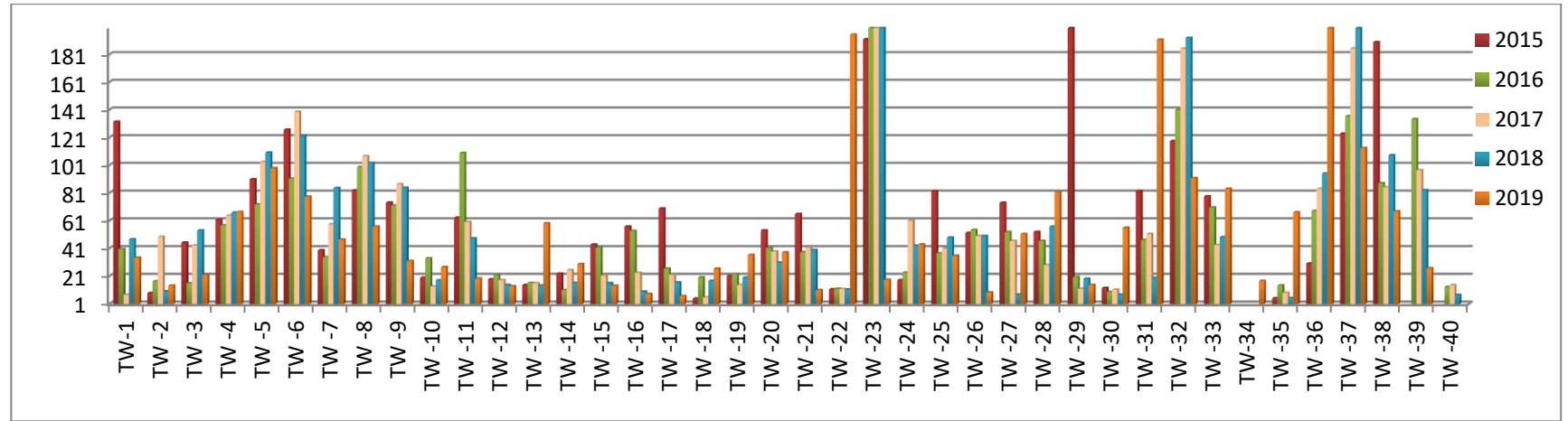
الشكل رقم (6-33): المعدلات السنوية لتركيز النيتروجين الكلي (N-T) في محطات التنقية خلال الأعوام (2014-2018)
