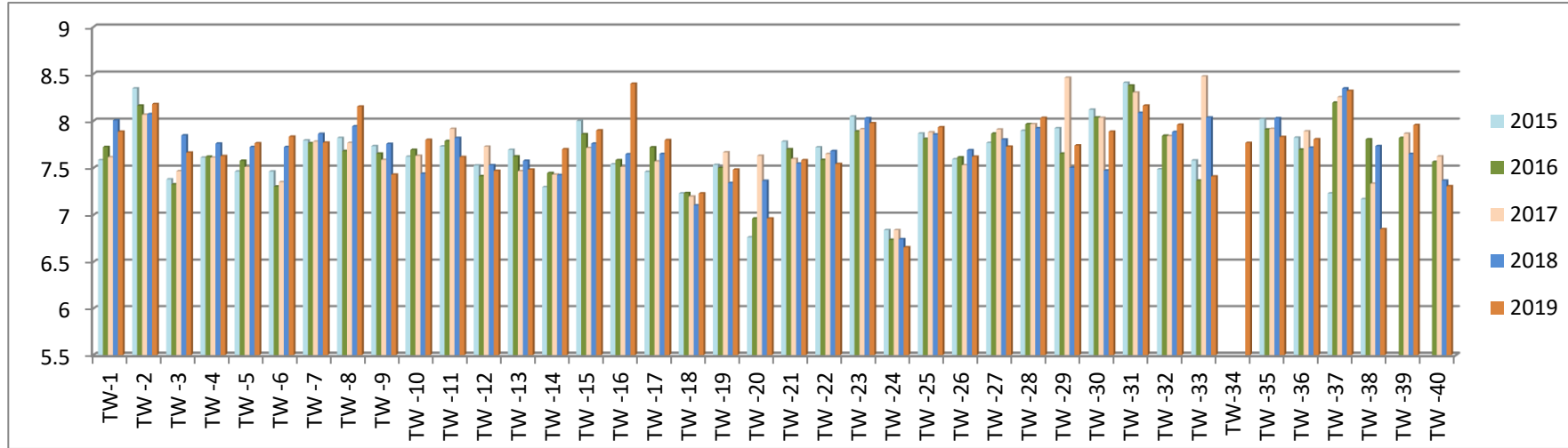
الشكل رقم (6-31): المعدلات السنوية لدرجة الحموضة (pH SU) في محطات التنقية خلال الأعوام (2015-2019)
