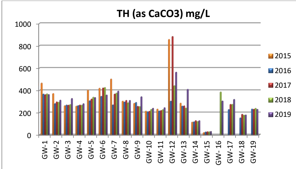
الشكل رقم (2-20): المعدلات السنوية لتركيز العسر الكلي (TH (as CaCO 3 ) mg/l) في مواقع المياه الجوفية خلال الأعوام (2015-2019)
