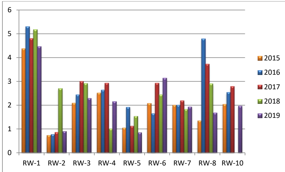
الشكل رقم (3-15): المعدلات السنوية لنسبة إدمصاص الصوديوم (SAR) في مياه السدود خلال الأعوام (2015-2019)
