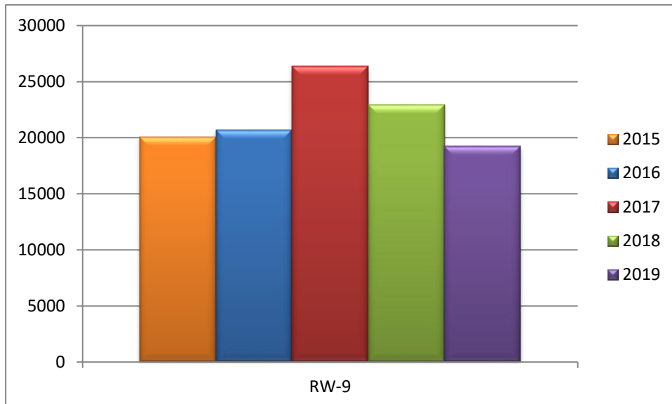
الشكل رقم (3-14): المعدلات السنوية لتركيز المواد الصلبة الذائبة الكلية في مياه سد الكرامة خلال الأعوام (2019-2015) (TDS mg/l)
