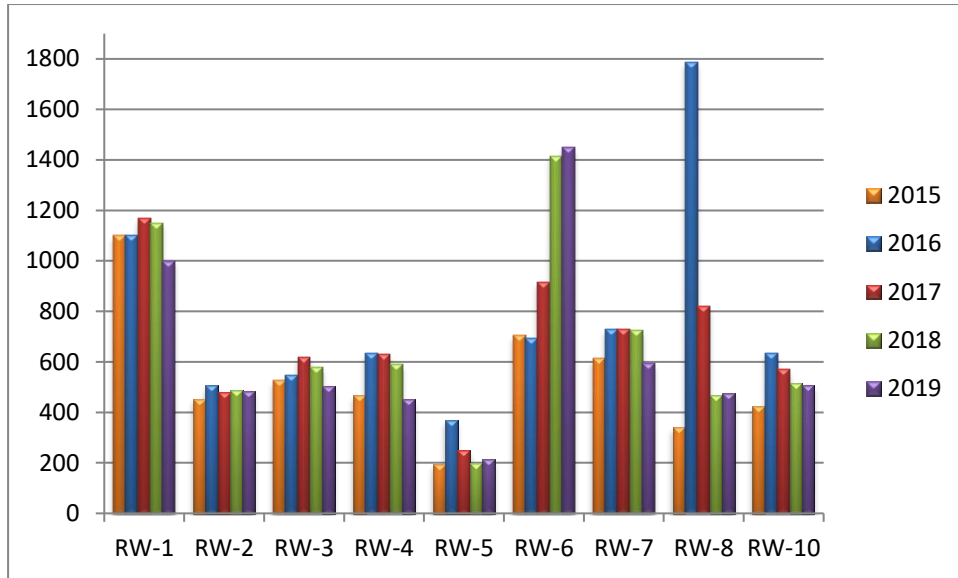
الشكل رقم (3-13): المعدلات السنوية لتركيز المواد الصلبة الذائبة الكلية في مياه السدود خلال الأعوام (2015-2019) (TDS mg/l)
