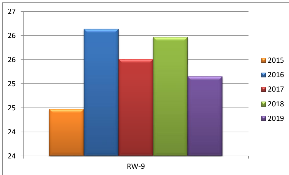
الشكل رقم (3-16): المعدلات السنوية لنسبة إدمصاص الصوديوم (SAR) في مياه سد الكرامة خلال الأعوام (2015-2019)
