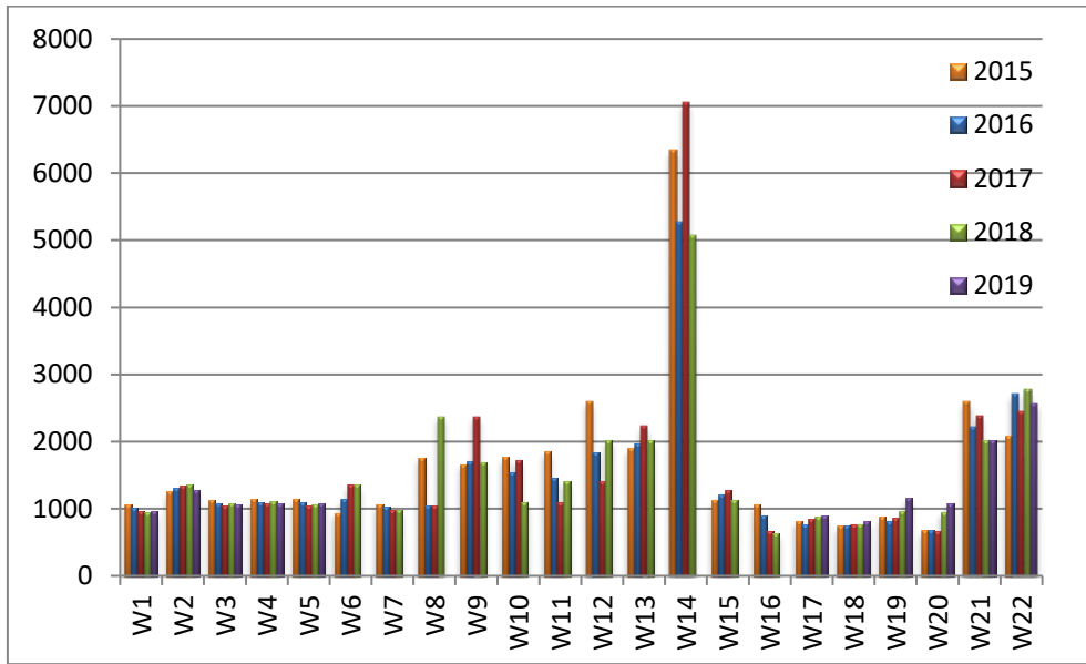
الشكل رقم (4-18): المعدلات السنوية لدرجة الملوحة (EC µS/cm) في مياه السيول والأودية خلال الأعوام (2015-2019)
