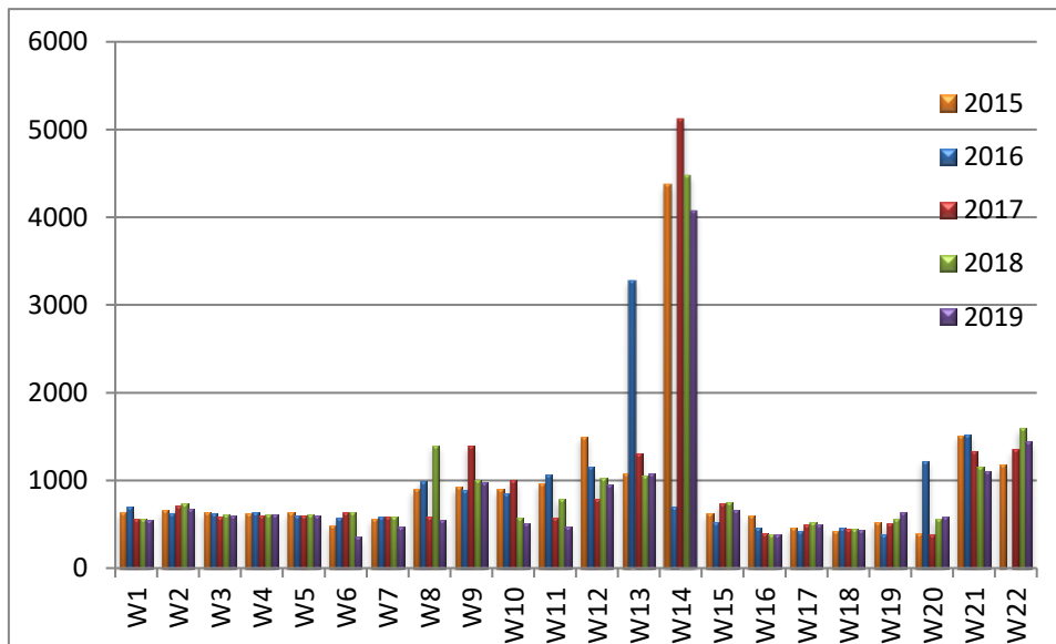
الشكل رقم (4-19): المعدلات السنوية لتركيز المواد الصلبة الذائبة الكلية (TDS mg/l) في مياه السيول والأودية خلال الأعوام (2015-2019)
