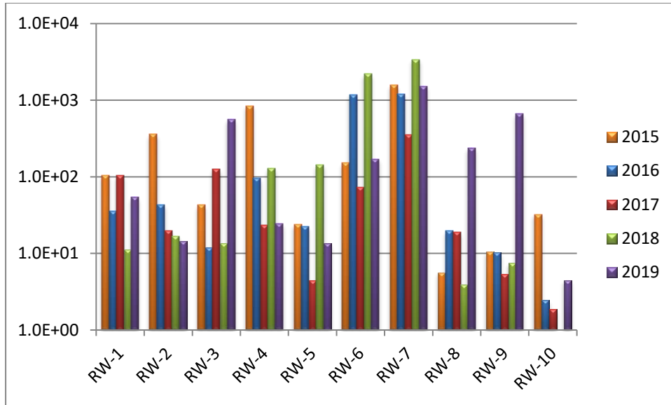
الشكل رقم (3-17): المعدلات الهندسية السنوية لأعداد الإشيرشيا القولونية ( E.coli MPN/100ml) في مياه السدود خلال الأعوام (2015-2019)
