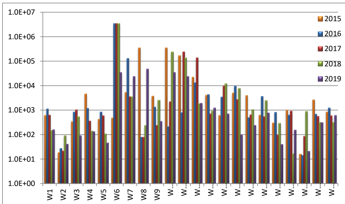
الشكل رقم (4-21): المعدلات الهندسية السنوية لأعداد الإشيرشيا القولونية ( E. coli MPN/100ml) في مياه السيول والأودية خلال الأعوام (2015-2019)
