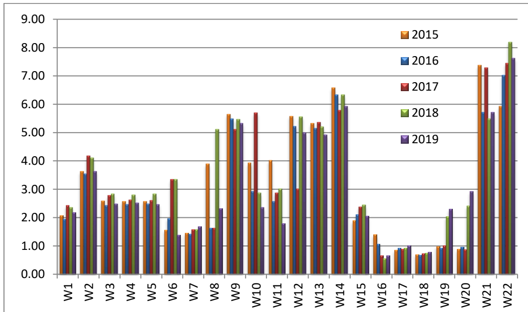
الشكل رقم (4-20): المعدلات السنوية لنسبة إدمصاص الصوديوم (SAR) في مياه السيول والأودية خلال الأعوام (2015-2019)
