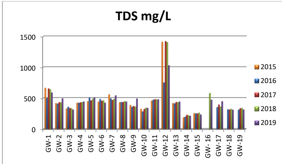
الشكل رقم (2-18): المعدلات السنوية لتركيز المواد الصلبة الذائبة الكلية (TDS mg/L) في مواقع المياه الجوفية خلال الأعوام (2015-2019)
