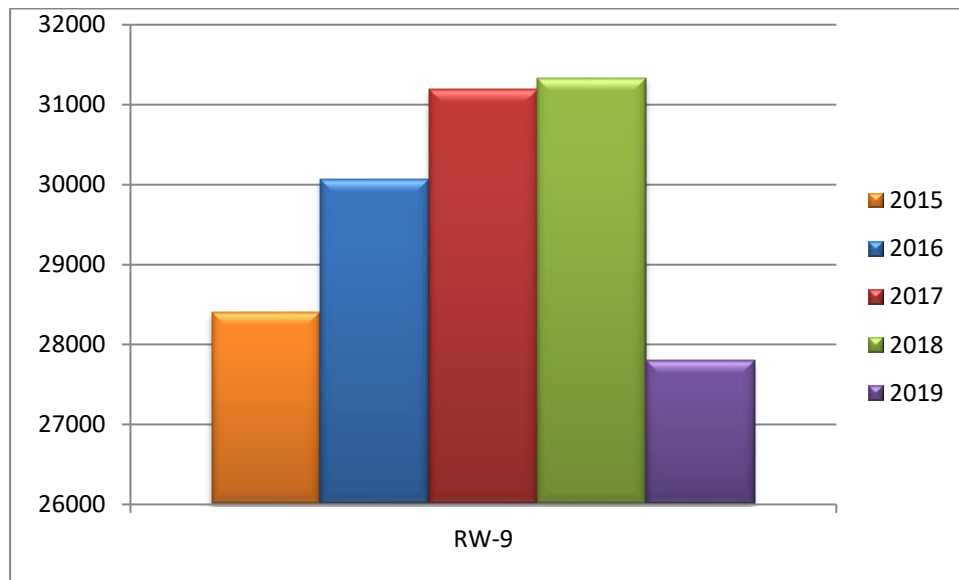
الشكل رقم (3-12): المعدلات السنوية لدرجة الملوحة (EC µS/cm) في مياه سد الكرامة خلال الأعوام (2019-2015)
