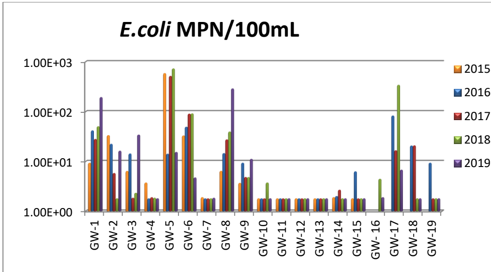
الشكل رقم (2-22): المعدلات الهندسية السنوية لأعداد الإشيرشيا القولونية ( E.coli MPN/100ml) في مواقع المياه الجوفية خلال الأعوام (2015-2019)
