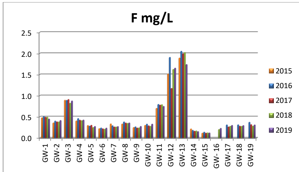
الشكل رقم (2-19): المعدلات السنوية لتركيز الفلوريد (F mg/l) في مواقع المياه الجوفية خلال الأعوام (2015-2019)
