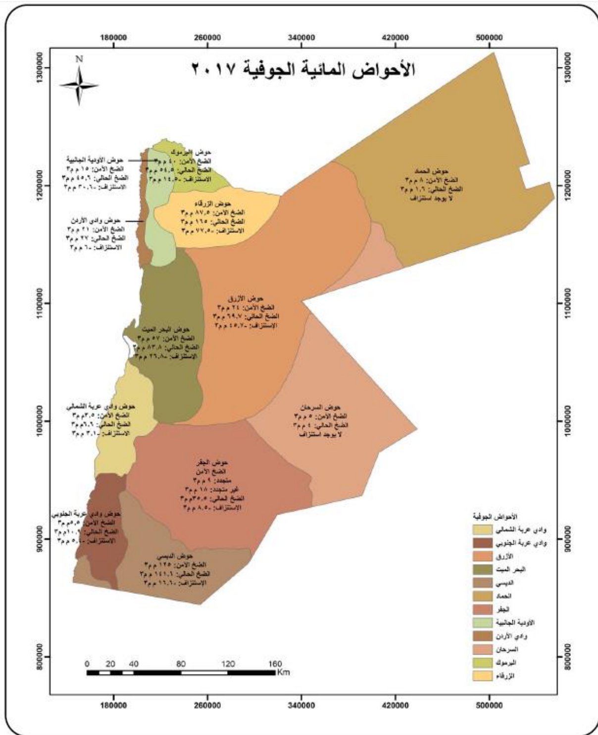
الشكل رقم (2-1): كميات الضخ والاستنزاف للأحواض المائية الجوفية لعام 2017 1
