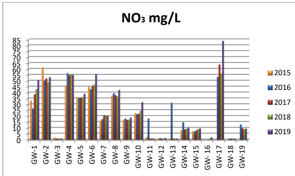
الشكل رقم (2-21): المعدلات السنوية لتركيز النترات (NO 3 mg/l) في مواقع المياه الجوفية خلال الأعوام (2015-2019)
